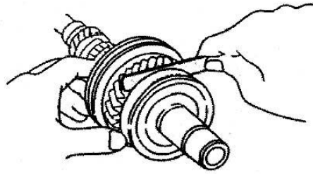
รูปที่ 10.8 แสดงการตรวจระยะห่างด้านข้างของแต่ละเฟืองเกียร์
