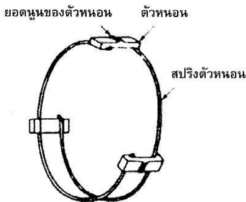
รูปที่ 10.6 แสดงตำแหน่งการตรวจความสูงของยอดนูนของตัวหนอนในชุดเฟืองซิงโครไนซ์
