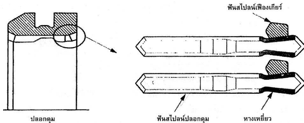
รูปที่ 10.9 แสดงการตรวจสอบการสึกหรอร่องทางเหยี่ยวของปลอกคুম
